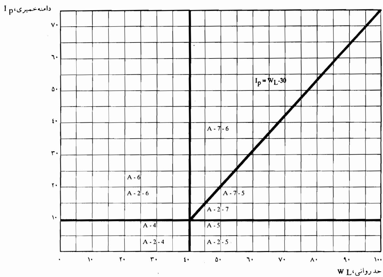
شکل (۱) محدوده حد روانی و دامنه خمیری خاکهای رس - لای دار
