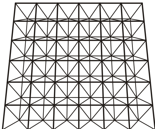
شکل ۳۷- شبکه دولایه با نقش دوراهه روی دوراهه (در سازه‌های دولایه در این پیوست، لایه بالا با خط کلفت تر و لایه پایین و جان با خط نازک تر نشان داده شده‌اند)
