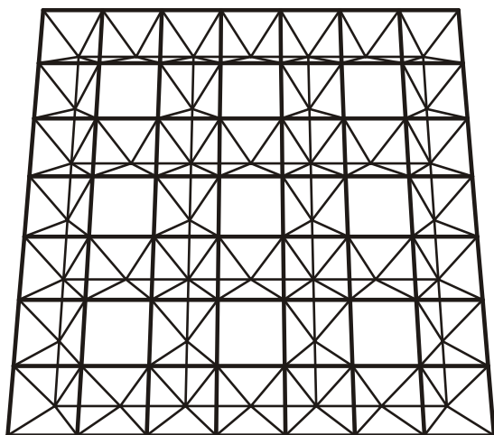
شکل ۳۹- شبکه دولایه با نقش دوراهه روی دوراهه بزرگتر
