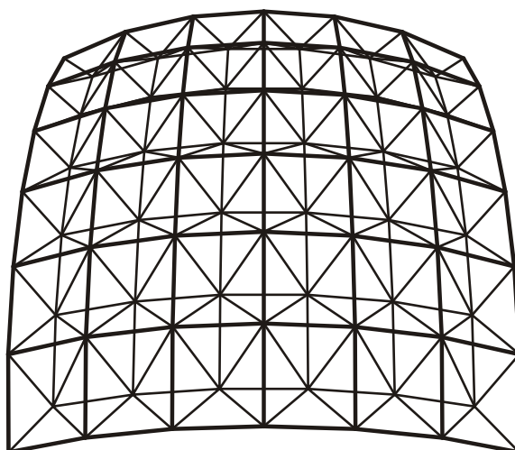
شکل ۱۴۰- گنبد دولایه فرازشی (کروی) با نقش دوراچه روی دوراچه
