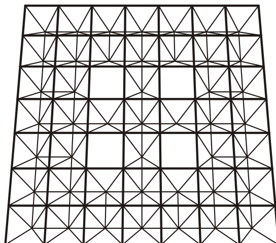
شکل ۳۸- شبکه دولایه با نقش دوراهه روی دوراهه و با چند چشمه باز
