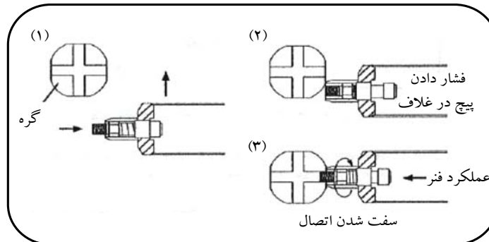
شکل (۱۵) : نحوه مونتاژ عضو به پیونده
