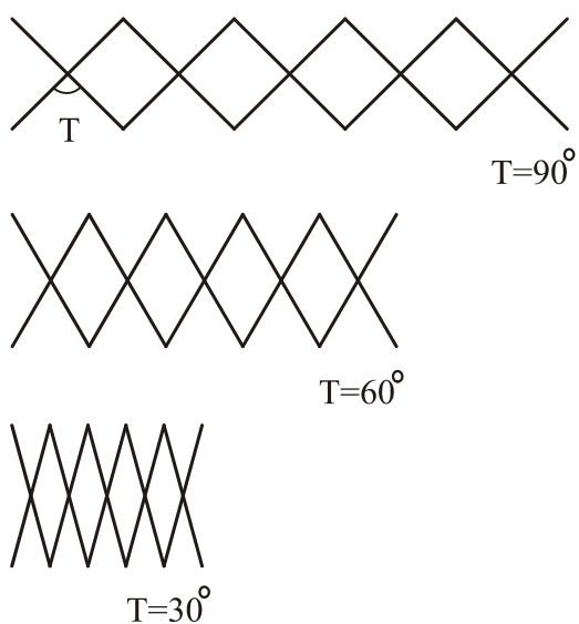
شکل ۱۹۸- یک سیستم ساده تاشو متشکل از پنج دولایه (سه حالت بازشدگی سیستم نشان داده شده است)
