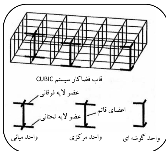
شکل (۴۱) : واحدهای سیستم CUBIC
