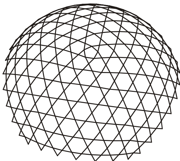
شکل ۱۴۴- گنبد ژئودزیک (بر مبنای ۵ رخ یک بیست رخ)
