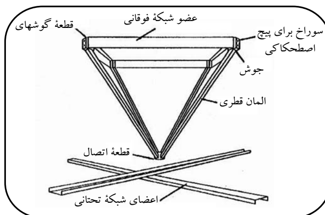
شکل (۳۹): جزئیات هر واحد سیستم UNIBAT
