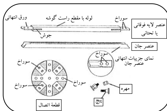
شکل (۲۴): قسمت های اصلی سیستم KETRUS
