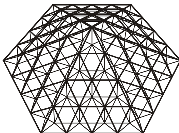
شکل ۱۷۹- هرم دولایه با قاعده شش بری
