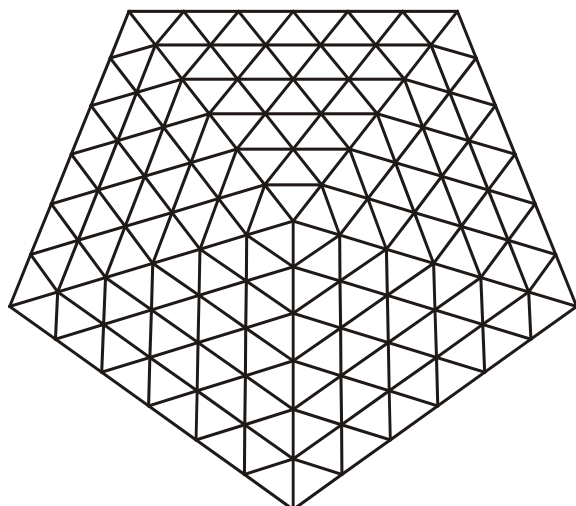
شکل ۱۸- شبکه قاچی تک لایه با نقش سه راهه
