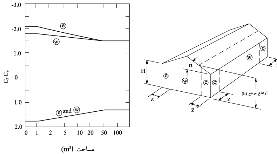
شکل ۹-۳- حداکثر ضریب خارجی C_p C_g در دیوارهای تک برای طراحی اجزای نمای ساختمان‌ها
