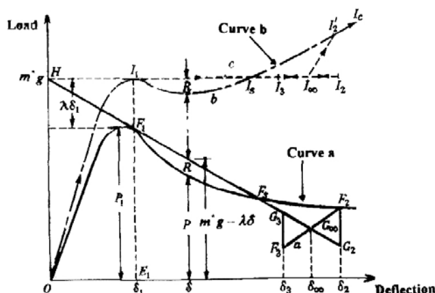
شکل ب-۵-۹- پاسخ بار- تغییر مکان خرابی ساده شامل یک عضو فشاری با اتصالات مفصلی
