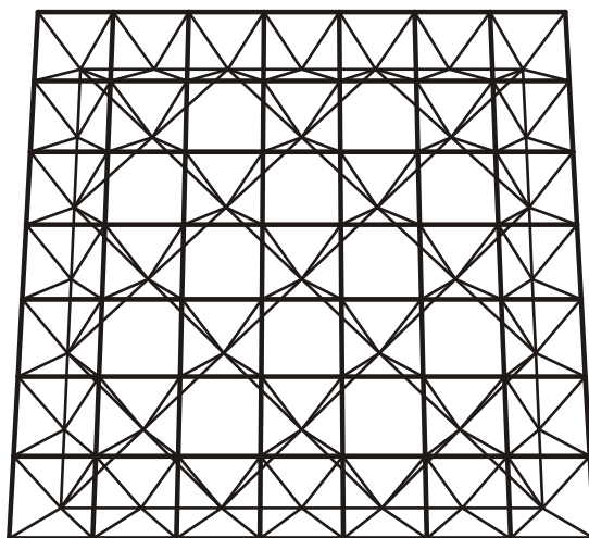
شکل ۴۷- شبکه دولایه با نقش دوراهه روی اریبی بزرگتر
