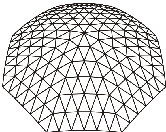
شکل ۱۳۹- گنبد قاچی فرازشی (ترکیب دو فرازش سهموی و مخروطی) با نقش سه‌راهه
