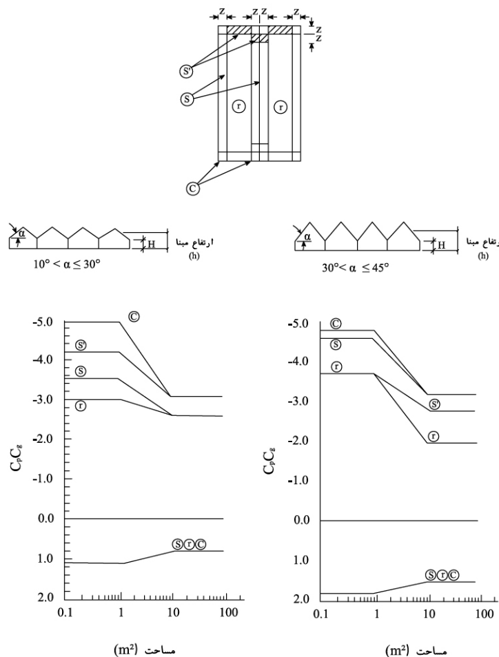
شکل ۳-۱۳ - ضرایب فشار خارجی C_p, C_g در سقف‌های شیروانی چند دهانه با شیب بزرگ‌تر از 10^\circ
