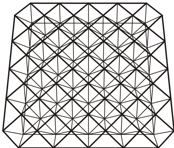
شکل ۴۳- شبکه دولایه با نقش اریبی روی اریبی
