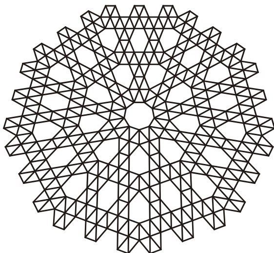
شکل ۲۵- شبکه قاجی تک لایه با نقش سه راهه / شش بری
