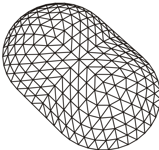
شکل ۱۶۱- چلیک-گنبد
