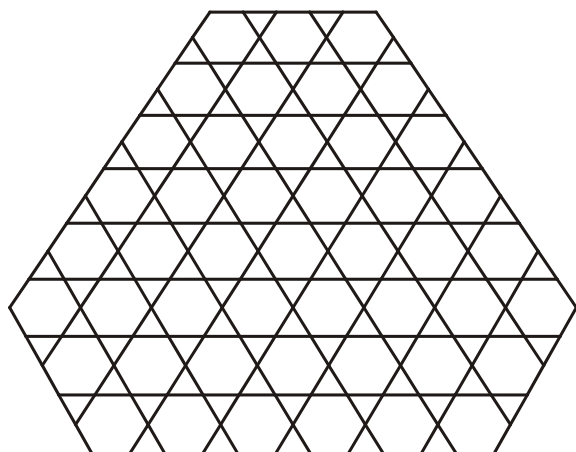
شکل ۱۶- شبکه مثلثی تک لایه با نقش سه راهه/شش بری و گوشه های بریده
