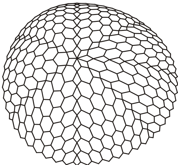
شکل ۱۰۹- گنبد تخم‌مرغی با ضرایب ۱/۱۵ و ۰/۸۵ برای مقیاس دو نیمه گنبد
