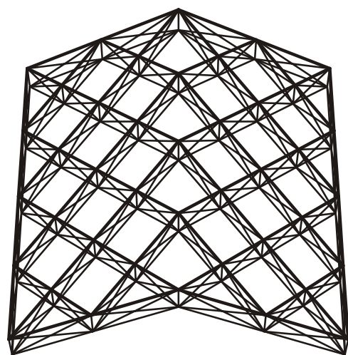
شکل ۹۰- چلیک لته ای دولایه فرازشی خریایی لملا
