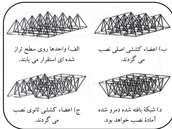
شکل (۳۸): مراحل مونتاژ سیستم SPACE DECK
