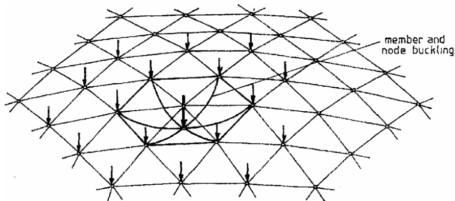
شکل پ-۴-۵- ناپایداری کوپل
