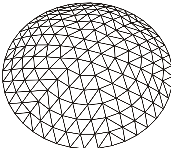
شکل ۱۰۴- گنبد دیامتیک
