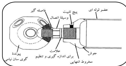
شکل ۶-۱۱: نمونه‌ای از سیستم‌های پیونده گوی‌سان
