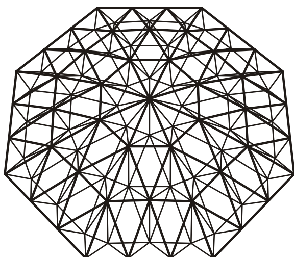
شکل ۱۴۱- گنبد قاچی دولایه فرازشی (سهموی) با نقش سه‌راهه روی سه‌راهه
