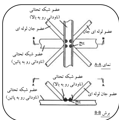
شکل (۴۴): جزییات سیستم HARLEY
