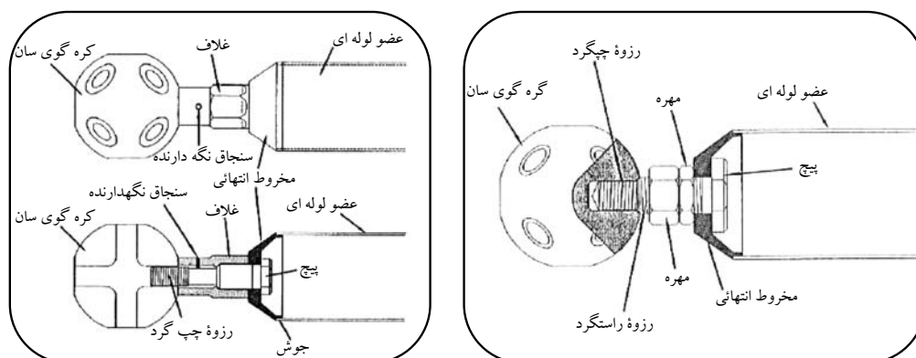
شکل (۱۲): سیستم ELKAR
