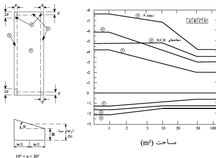
شکل ۳-۱۵- ضرایب فشار خارجی C_p, C_g برای سقف‌های دندانه‌ای با شیب 10^\circ و بیشتر
