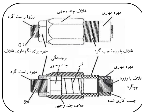
شکل (۱۴): جزئیات پیچ KT-TRUSS
