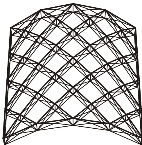
شکل ۸۹- چلیک سهموی دولایه فرازشی خریایی لملا
