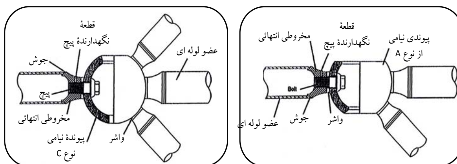
شکل (۱۸) : سیستم نیامی NS - نوع C
