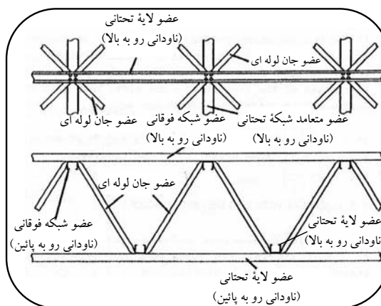
شکل (۴۳): سیستم HARLEY
