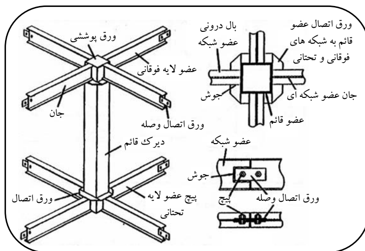
شکل (۴۲): جزییات هر واحد سیستم CUBIC
