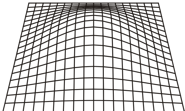
شکل ۱۴۸- گنبد نوانشی با نقش دوراهه و کناره‌های درجا نگهداشته (حالت ۳ نوانش به کار رفته است)
