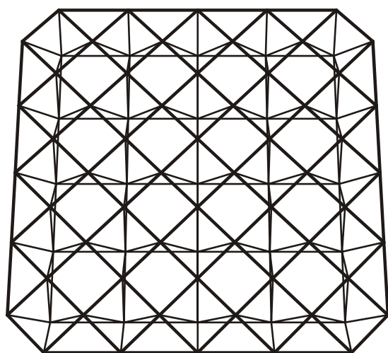
شکل ۴۸- شبکه دولایه با نقش اریبی روی دوراهه بزرگتر
