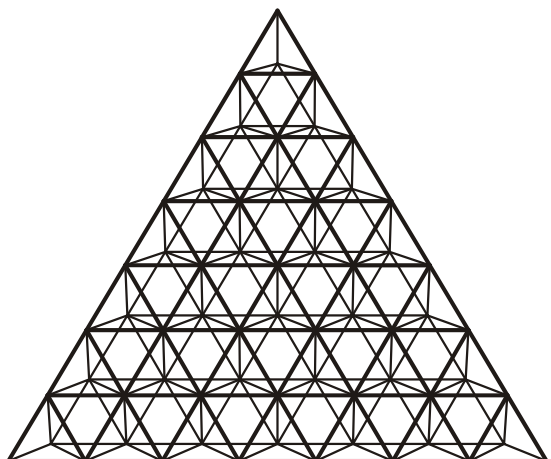
شکل ۵۵- شبکه دولایه با نقش سه راهه روی سه راهه و پلان مثلثی
