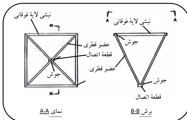
شکل (۳۶): جزییات هر واحد سیستم SPACE DECK
