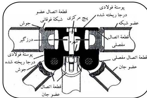
شکل (۳۴) : سیستم NODUS
