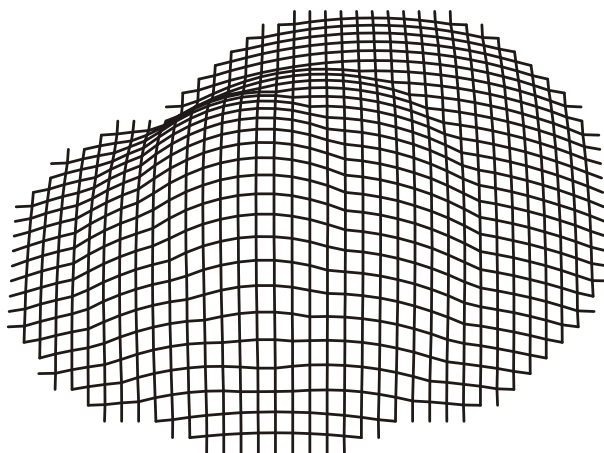
شکل ۱۸۵- شکل آزاد: شبکه تک لایه فرازیده با نقش دوراهه (۳ فراش سهموی به کار رفته است)
