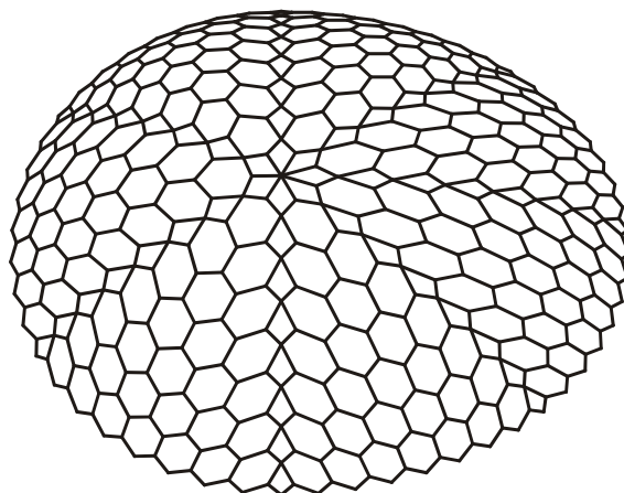
شکل ۱۱۰- گنبد تخم‌مرغی با ضرایب ۱/۳۵ و ۱/۰۵ برای مقیاس دو نیمه گنبد
