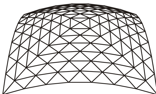
شکل ۱۵۲- گنبد قاچی نوانشی با نقش سه‌راهه و گوشه‌های درجانه‌گذاشته (حالت ۳ نوانش و یک نقطه مرکزی برآمده به کار رفته است)
