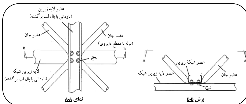
شکل ۶-۸: نمونه‌ای از اتصال پرسی
