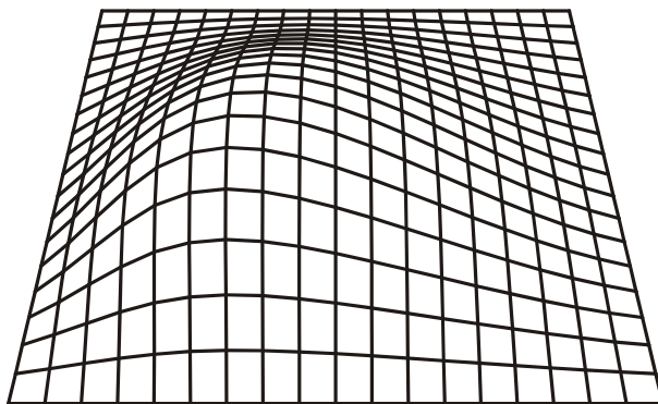
شکل ۱۴۹- گنبد نوانشی با نقش دوراهه و کناره‌های درجا نگهداشته (حالت ۳ نوانش به کار رفته است)
