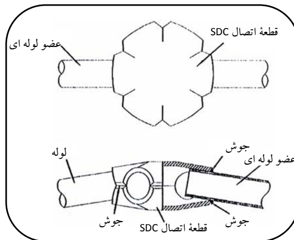
شکل (۳۵) : سیستم SDC
