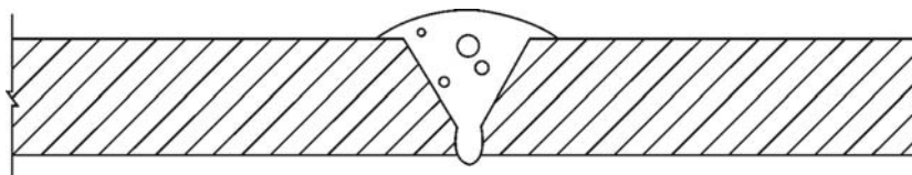
شکل ۱۷-۵-۶-۵-۲ ب تخلخل در جوش.
