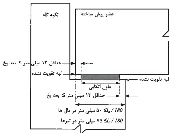
شکل ۹-۱۷-۵ حداقل ابعاد در اتصالات اتکایی
