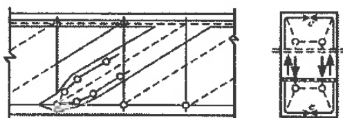
پ- عضو فشاری قطری در جابجایی خالص
