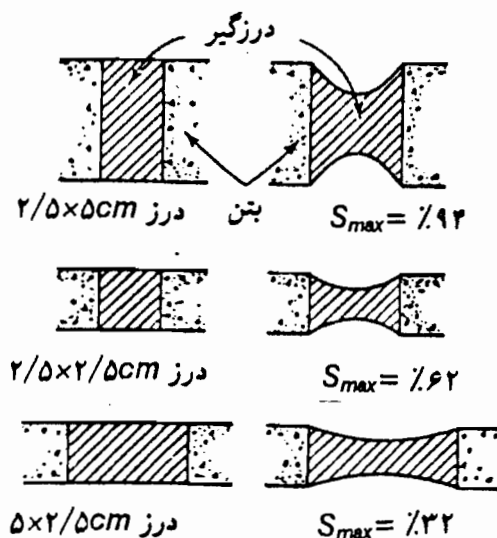
شکل ۴-۵- کرنش سطحی برای افزایش عرض 12/5 میلیمتر
