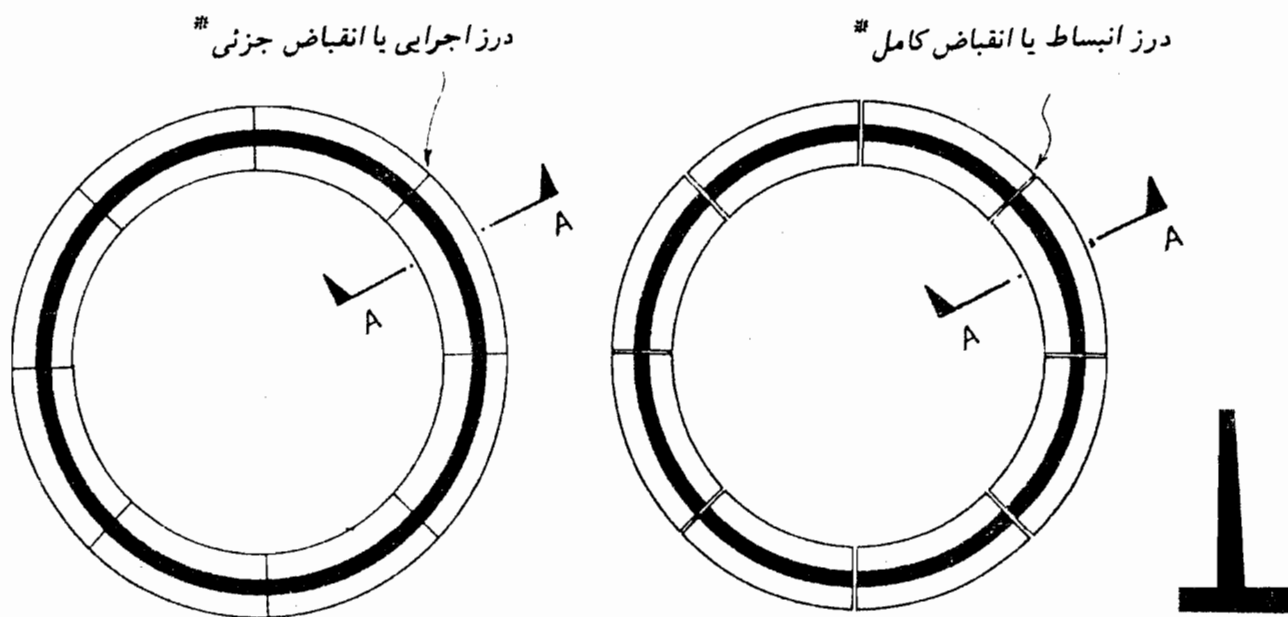
الف: پلان مخزن استوانه‌ای با دیوار یکپارچه
