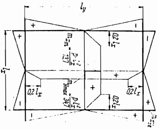
نمودار لنگر
