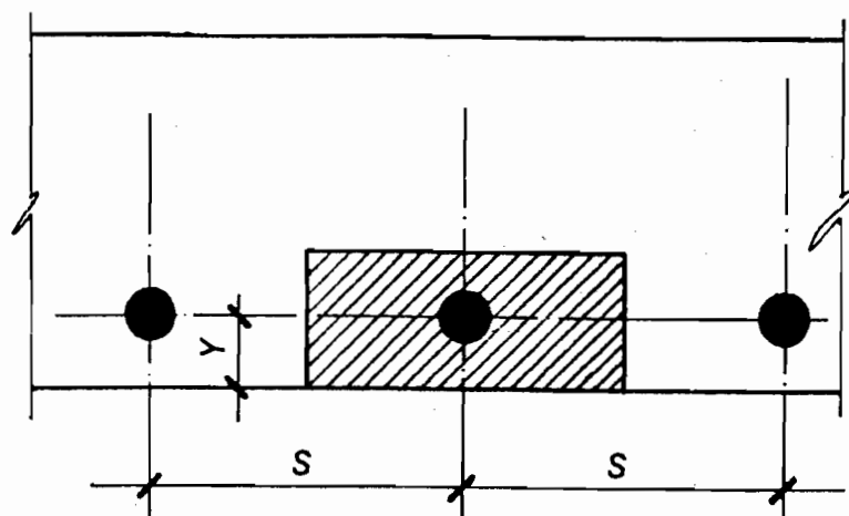
الف: دال‌ها
