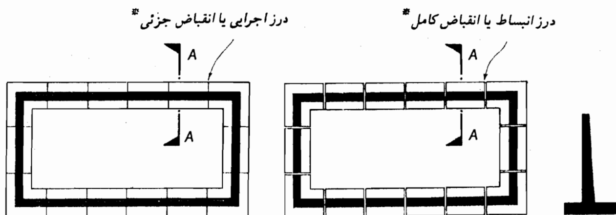
الف: پلان مخزن مستطیلی با دیوار یکپارچه
