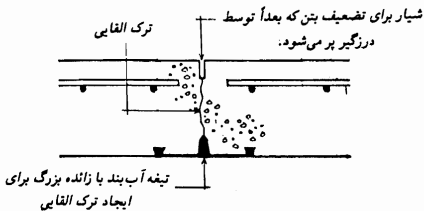
شکل ۴-۶- درز انقباض القایی
