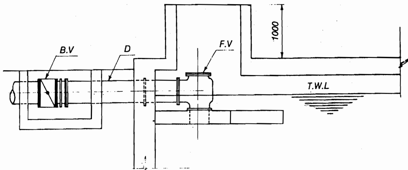
مقطع
