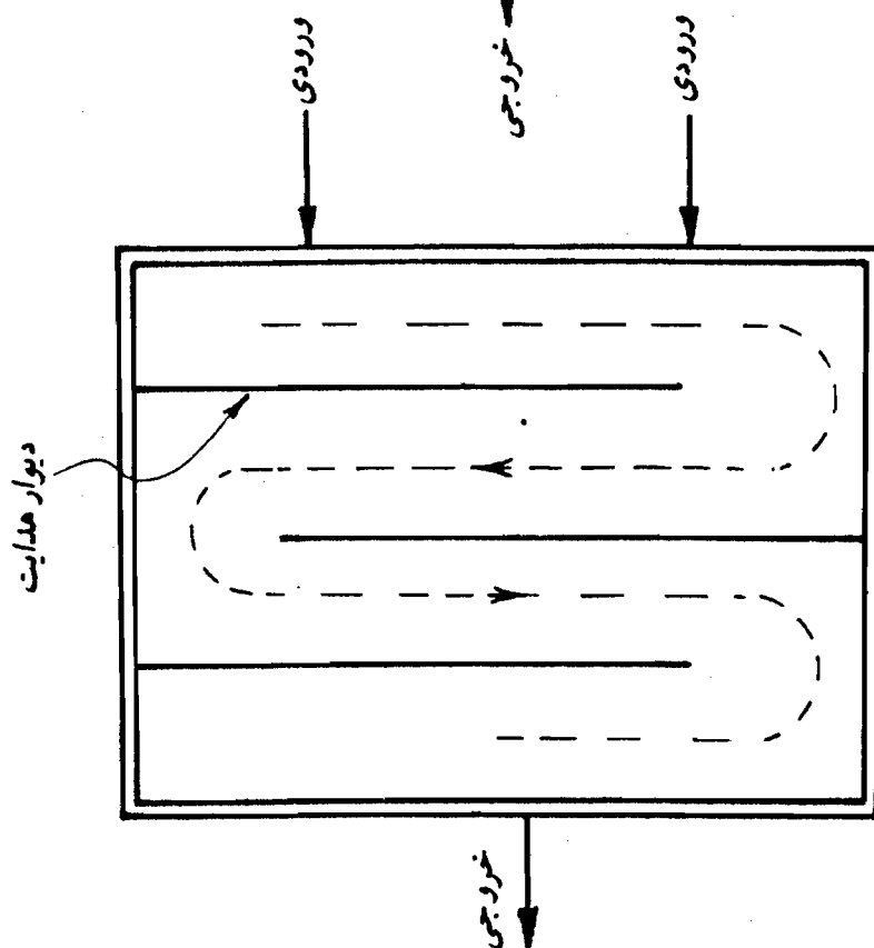
الف: مخازن کوچک و متوسط
