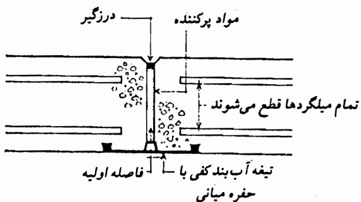
شکل ۴-۷- درزهای انبساطی
