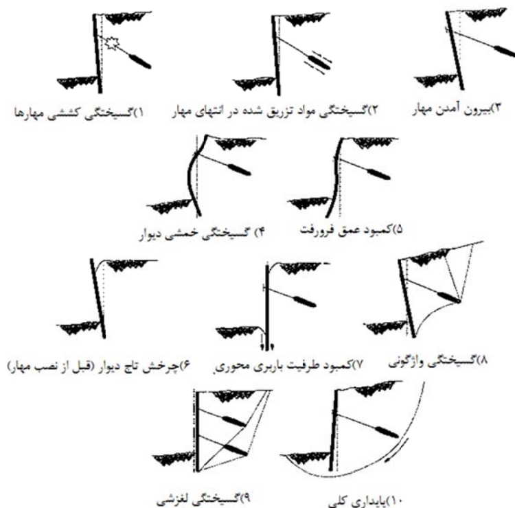
شکل ۷-۱-۵-۷ حالت‌های حدى دیوارهای مهار شده
